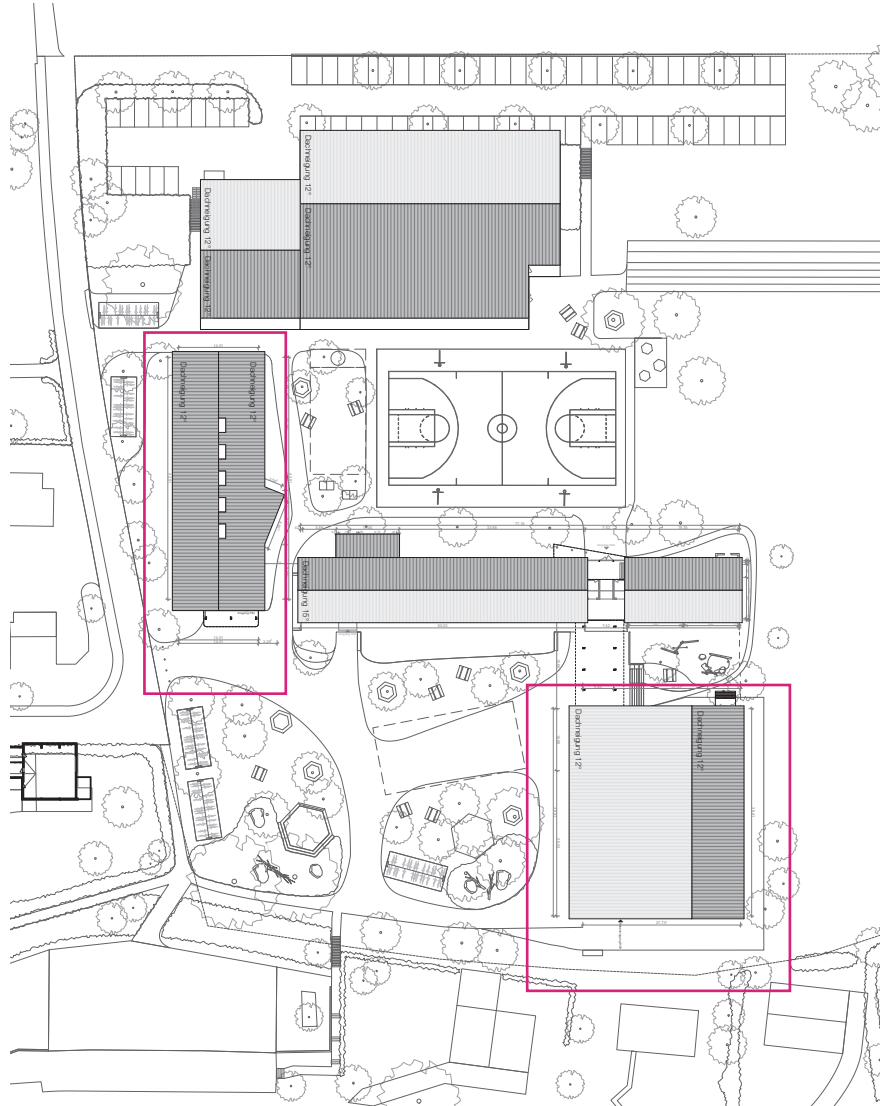
Abb. 2 Vorprojekt Dachaufsicht mit neuen Gebäudevolumen pink umrahmt, Schmid Schärer Architekten
